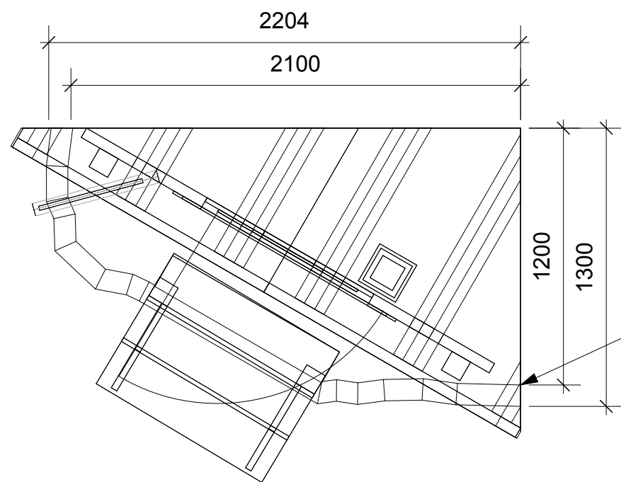
01 Oaken Sauna Top Scale 1:25
