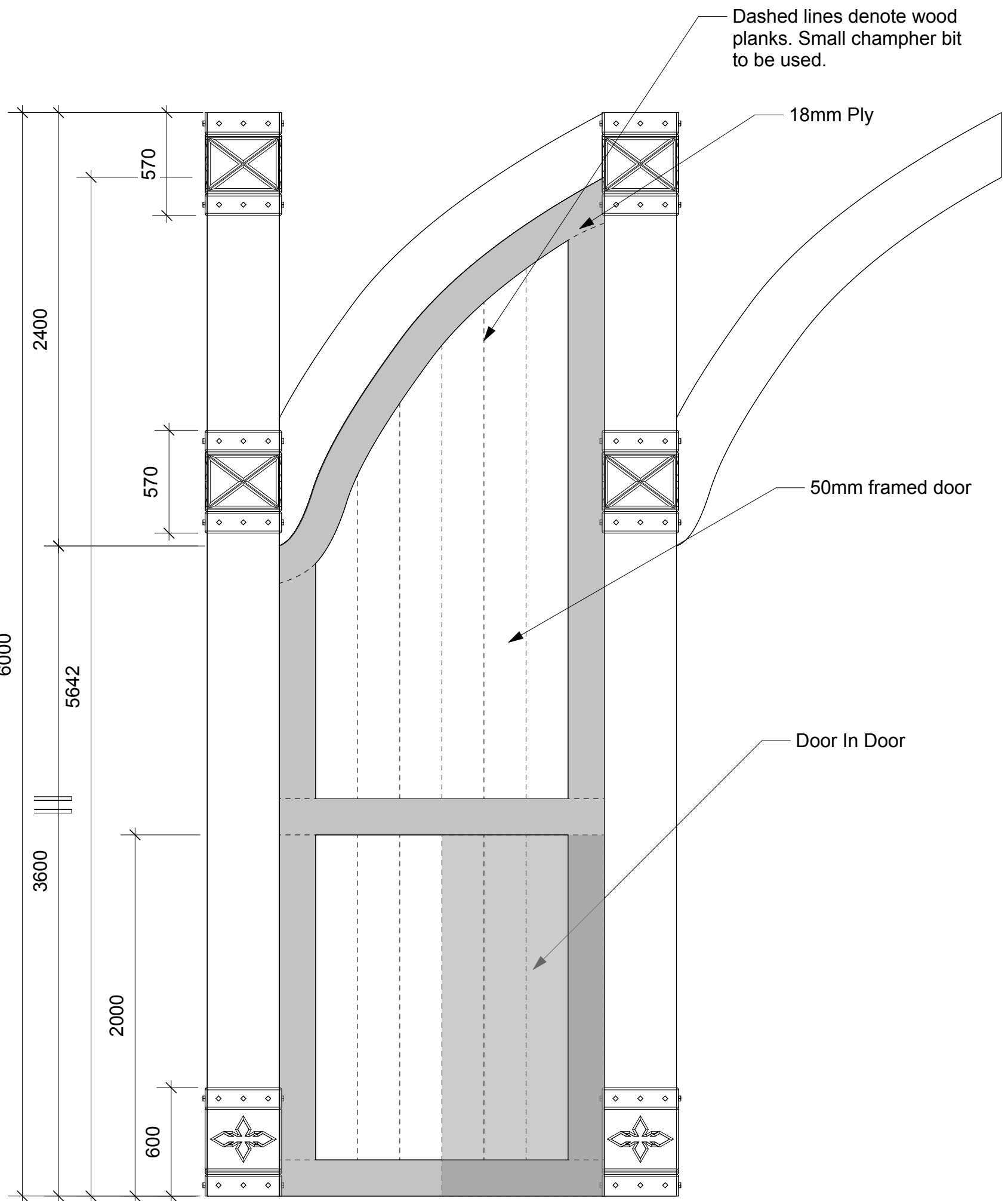
01 Door & Arch Front Scale 1:25
