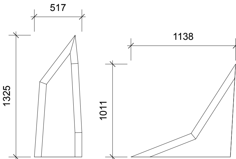
03 Ice Palace OP Layer 3 Scale 1:25
